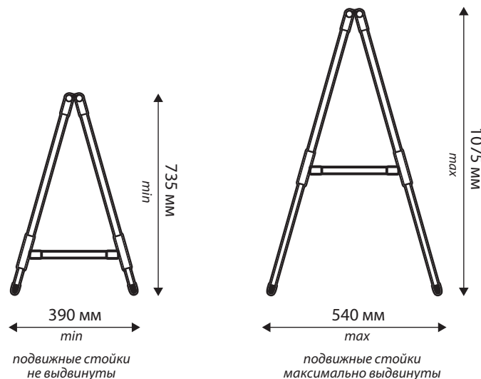
Рис. 2 Размеры мольберта
