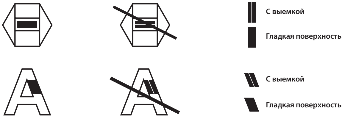
Рис. 3 Схема установки магнитов.
