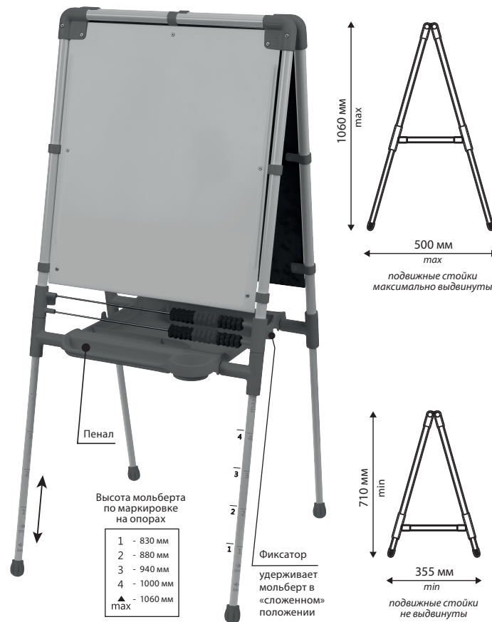
Рис. 1 Мольберт в рабочем положении
